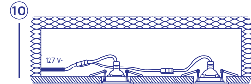
Diagrama para instalar una lámpara a 127 V - Diagram to install a lamp at 127 V -
