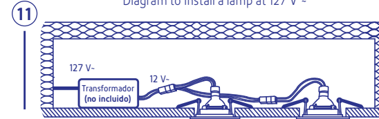
Diagrama para instalar una lámpara a 12 V - Diagram for installing a lamp at 12 V -
